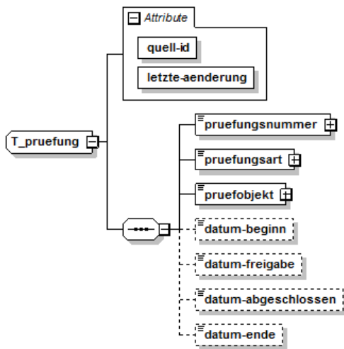
Abbildung 23: XML-Struktur T_pruefung
