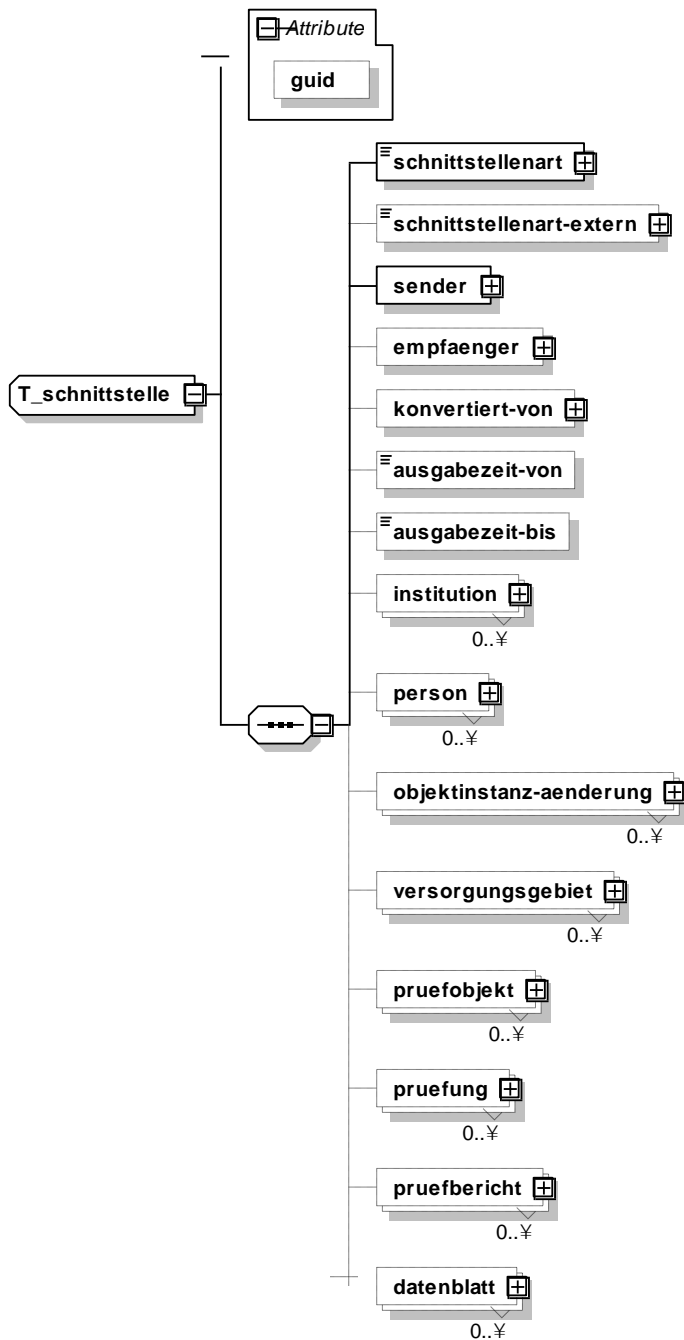
Abbildung 5: XML-Struktur T_schnittstelle
