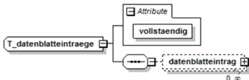
Abbildung 1: XML-Struktur T_datenblatteintraege
