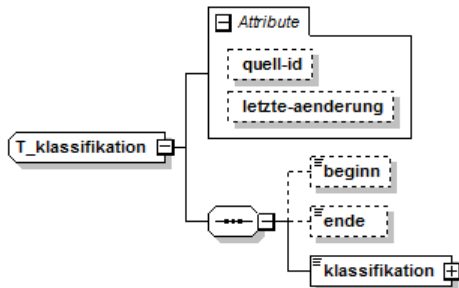
Abbildung 22: XML-Struktur T_klassifikation
