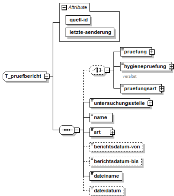
Abbildung 24: XML-Struktur T_pruefbericht
