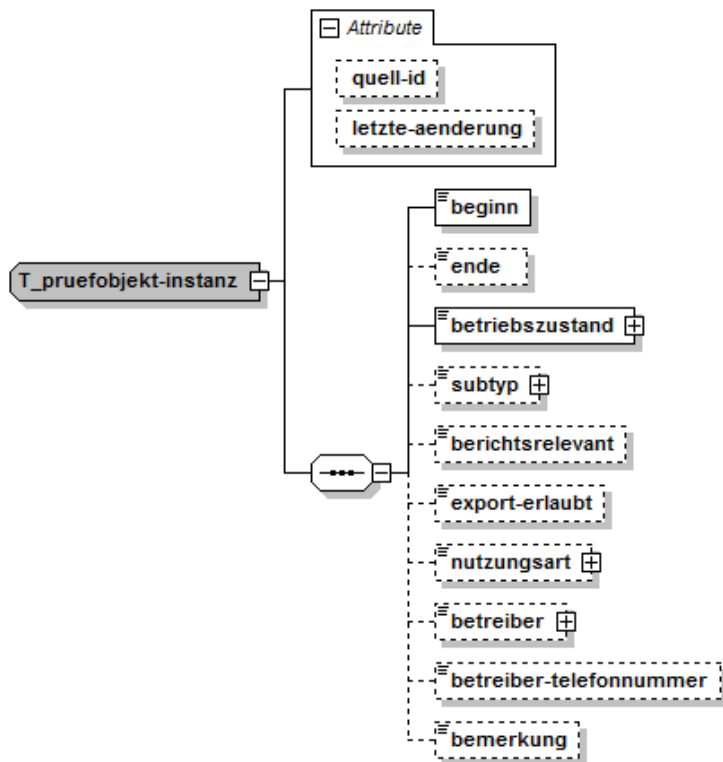
Abbildung 17: XML-Struktur T_pruefobjekt-Instanz
