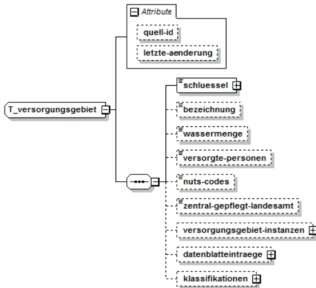
Abbildung 10: XML-Struktur T_versorgungsgebiet
