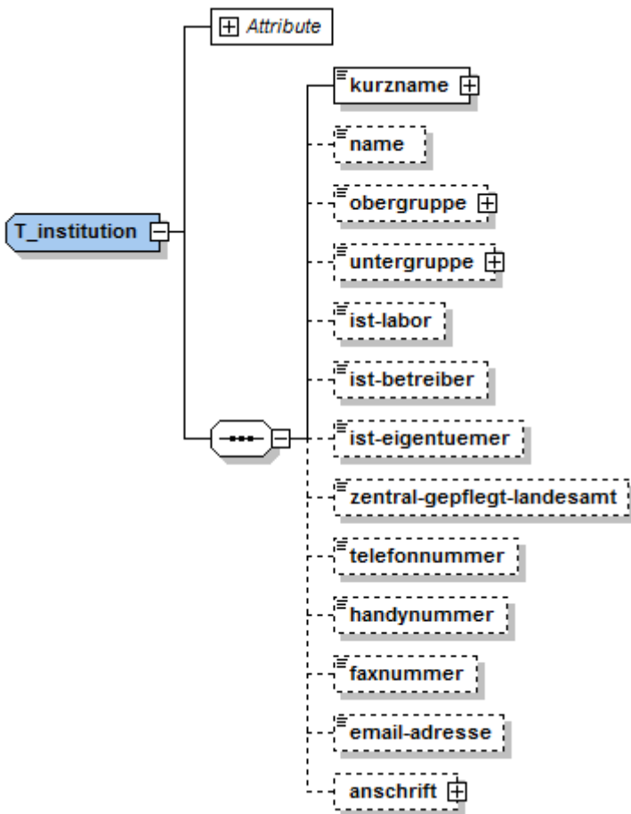
Abbildung 8: XML-Struktur T_institution
