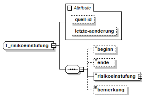
Abbildung 19: XML-Struktur T_risikoeinstufung
